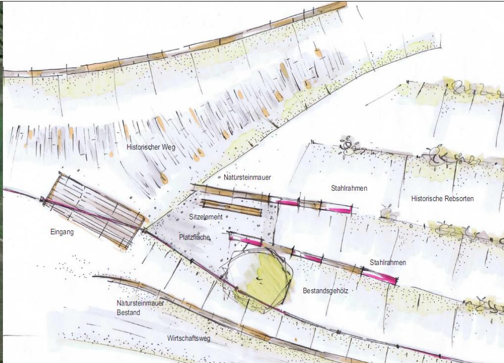
Entwurfsskizze: Lageplan südliche Platzfläche
